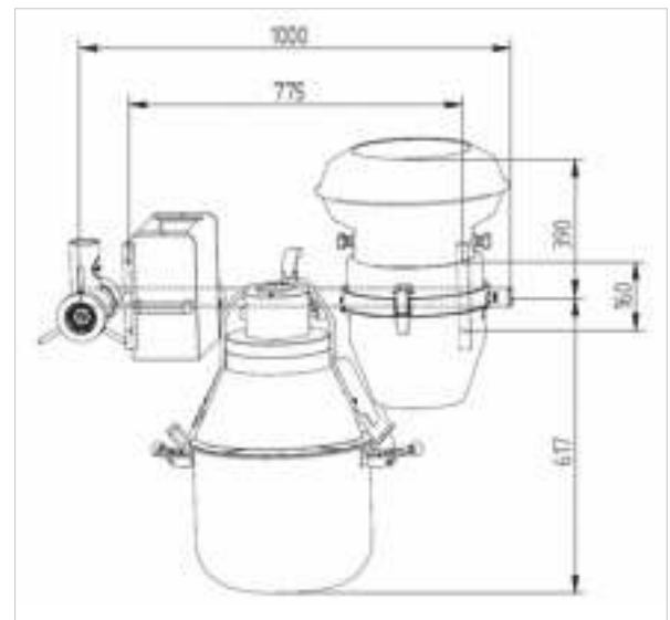
Wandleiste Geräteaufnahmen
